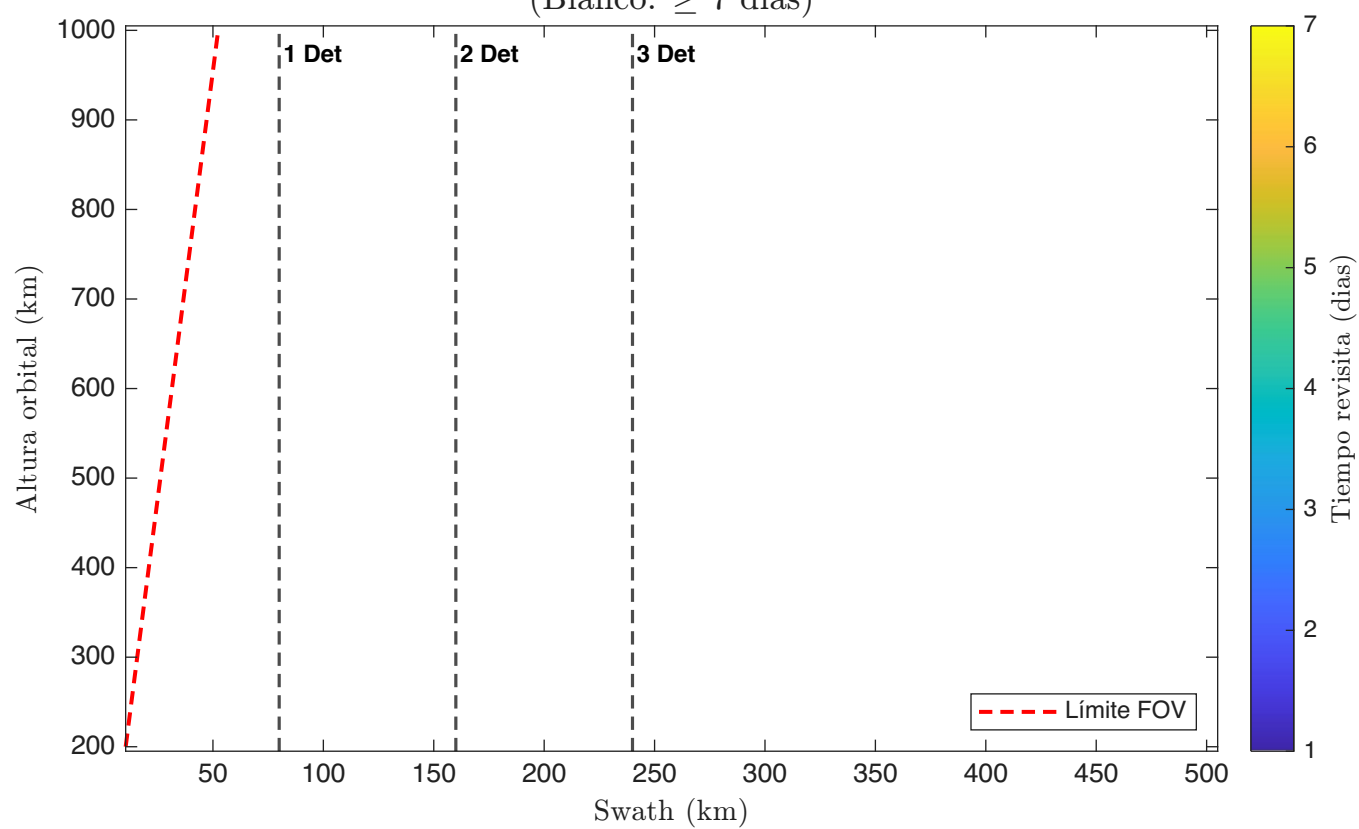
Tiempo Revisita - 2 Satellite(s); 1 Telescopio(s): Cassegrain; Detector 3 (Blanco: \geq 7 dias)
